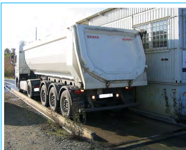
Foto: Brückenwaage mit Seitenführung
