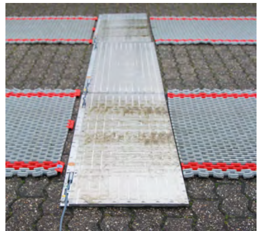
Die Auffahrt auf die Radlastwaagen zur Messung der Achslast muss in diesem Fall von rechts erfolgen, da der Kabeldurchlass für die Messkabel an der linken Ausgleichsmatte vorgesehen ist.
